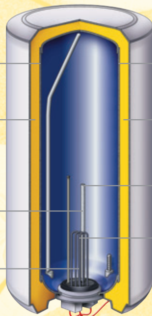
Schnitt Elektro-Wassererwärmer Coupe chauffe-eau blindé
