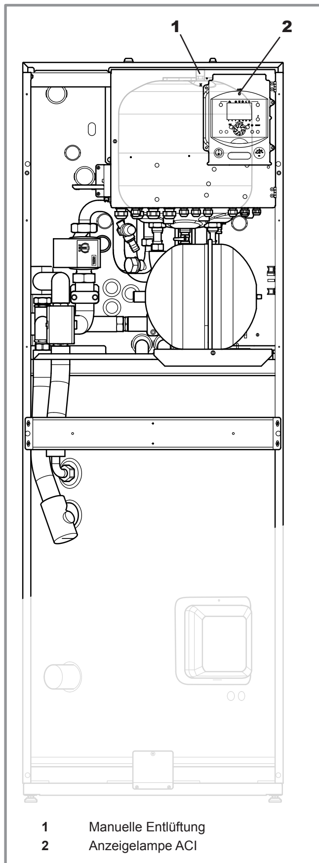
Abbildung 14 - Manuelle Entlüftung und Anzeigelampe ACI
